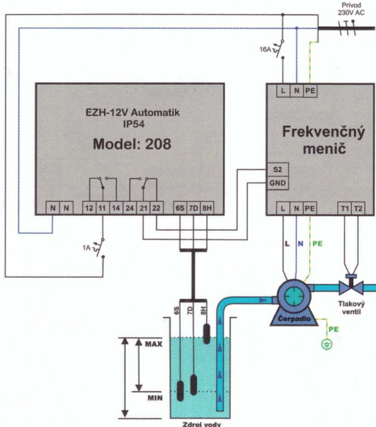
Zvýšenie ochrany pri použití frekvencného meniča
