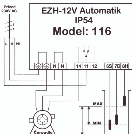
Príklad zapojenia: Model 116
